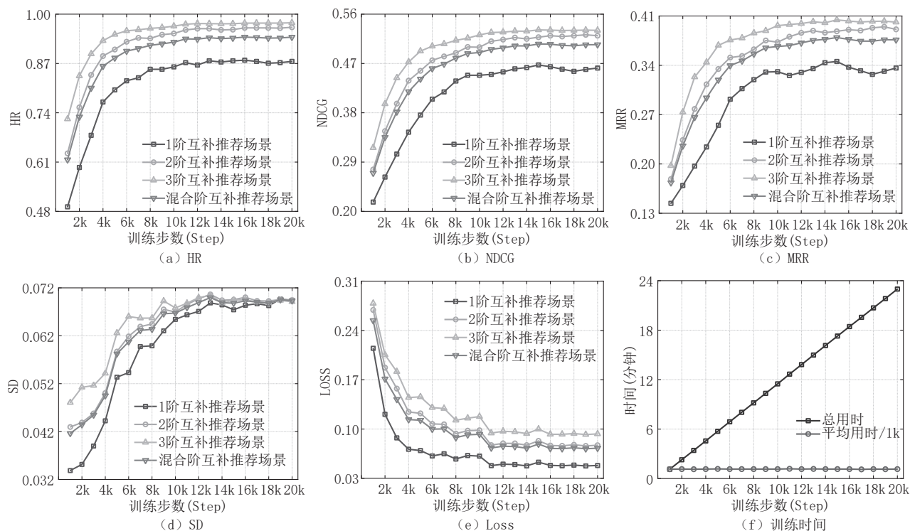
图11 PWA数据集下模型训练效果
