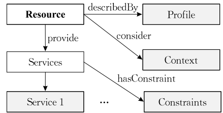
图 8 一种基于本体的物端资源和物理实体服务描述模型
