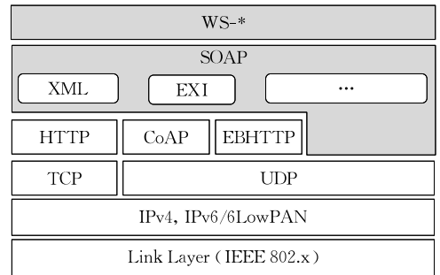
图 5 WS-based Web 风格的实体服务实现架构
