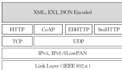
图 6 RESTful Web 风格的实体服务实现架构
