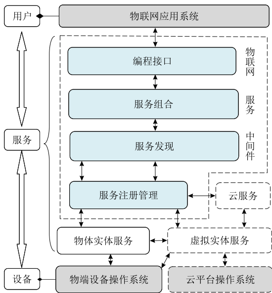
图2 面向服务的物联网服务中间件的功能模型
