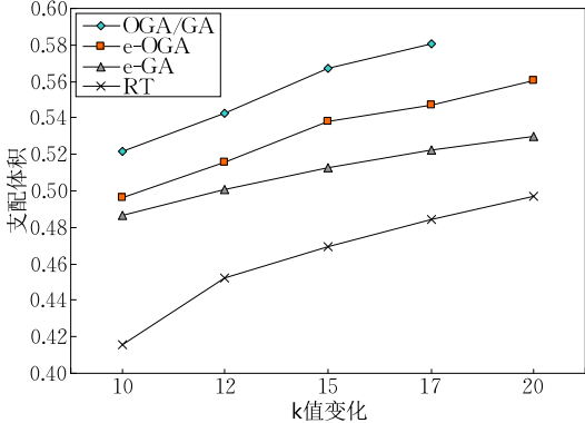
(b) 反相关数据集( \epsilon=0.1 )
