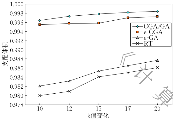
(a) 独立数据集( \epsilon=0.01 )
