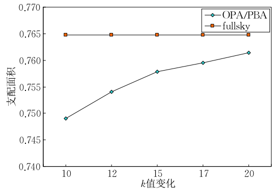
图 16 k 值变化对支配面积(支配体积)的影响
