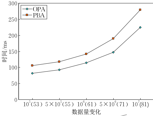
图 13 数据量变化对算法运行时间的影响
