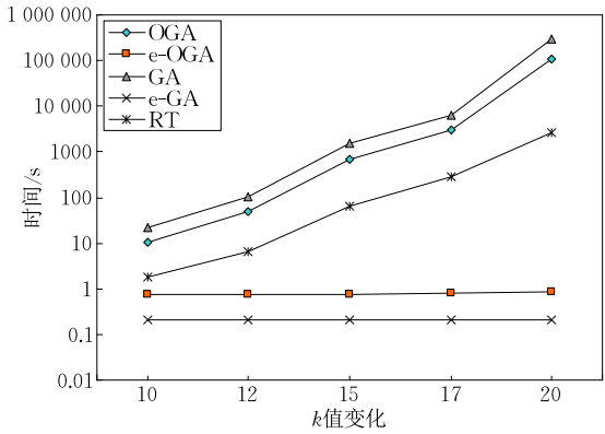
(a) 独立数据集( \epsilon=0.01 )
