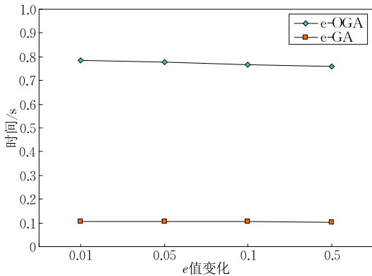
(a) 独立数据集
