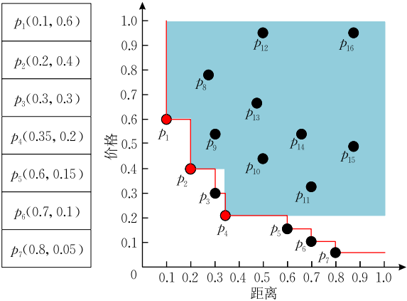
图 1 轮廓和 k 最大覆盖轮廓( k=3 )
