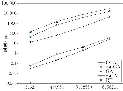
(a) 独立数据集( \epsilon=0.01 )
