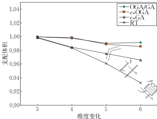
(a) 独立数据集( \epsilon=0.01 )
