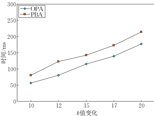
图 15 k 值变化对算法运行时间的影响
