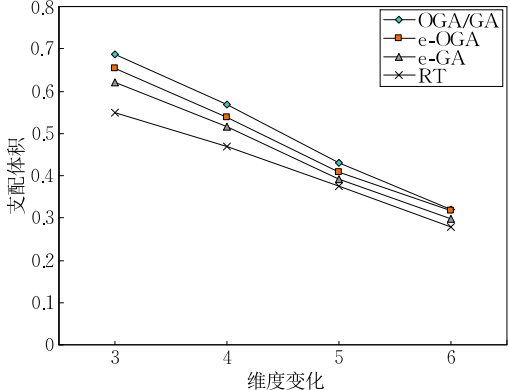
(b) 反相关数据集( \epsilon=0.1 )
