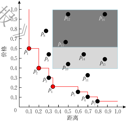
图 2 集合的支配大小举例
