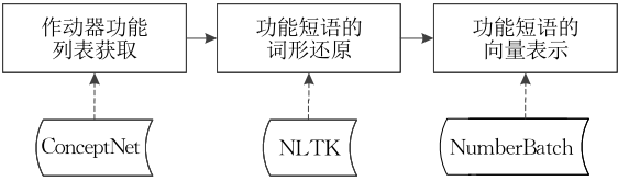
图 3 作动器功能列表获取与处理流程
