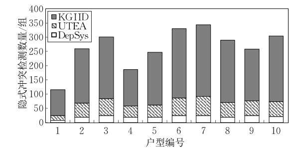
图 9 三种方法的隐式冲突检测数量对比
