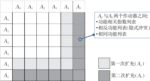
图7 隐式冲突矩阵
