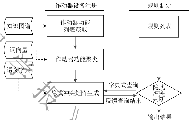
图1 KGIID方法整体流程
