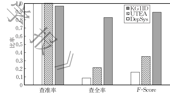
图 10 三种方法的查准率、查全率和 F -score 指标对比
