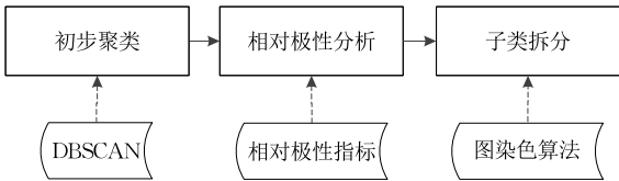
图 4 作动器功能聚类流程
