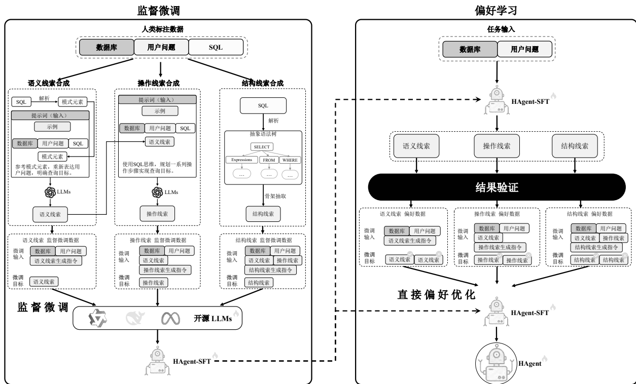
图 4 HAgent 两阶段微调框架
