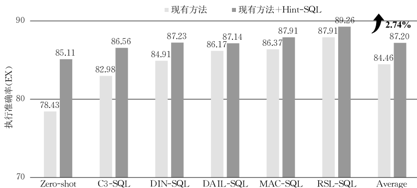
图 6 Spider 上的增强结果(使用 GPT-4o 模型)
