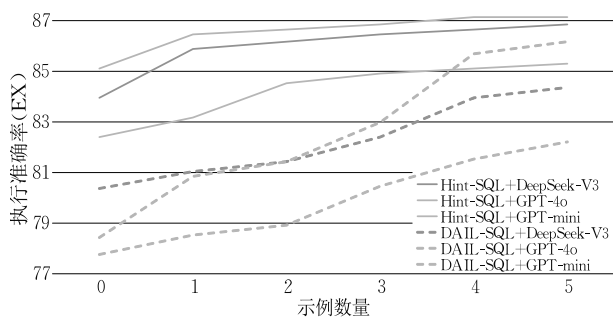
图 10 示例数量对结果的影响(Spider 数据集)
