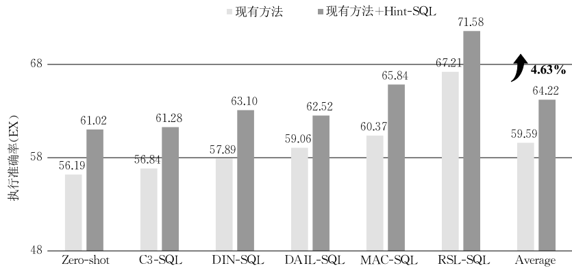
图 7 BIRD 上的增强结果(使用 GPT-4o 模型)
