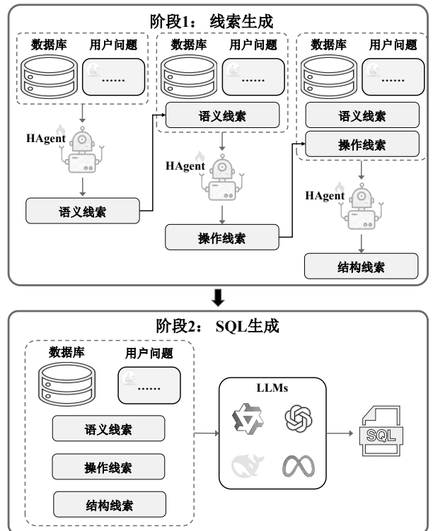
图 3 Hint-SQL 流水线示意图
