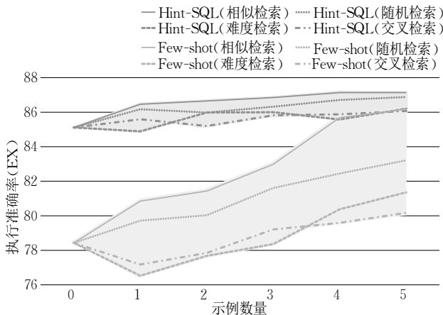
图 12 示例质量对结果的影响(Spider 数据集)
