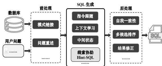
图 2 Text-to-SQL 三阶段流水线示意图
