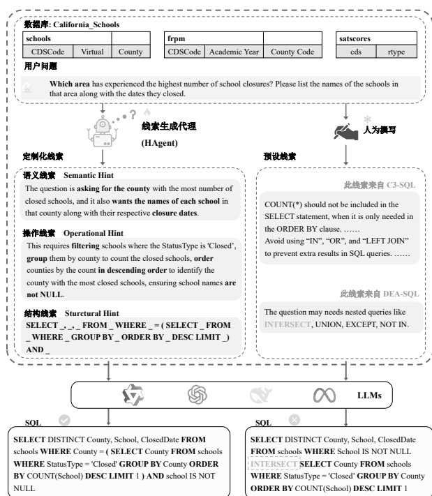
图 1 Hint-SQL 与现有方法的对比(省去了示例、任务指令等其他提示词内容)
