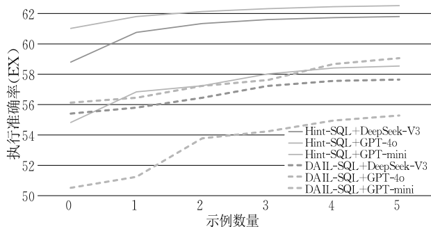
图 11 示例数量对结果的影响(BIRD 数据集)
