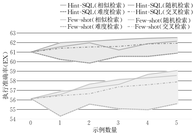
图 13 示例质量对结果的影响(BIRD 数据集)
