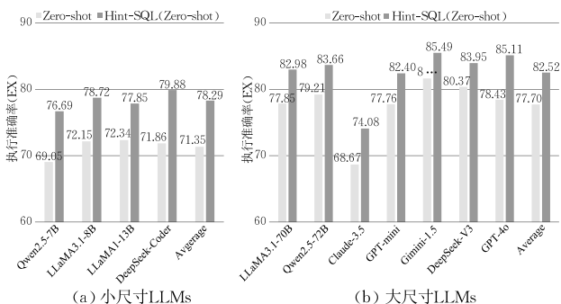
图 8 零样本场景下 Hint-SQL 的结果(Spider 数据集)
