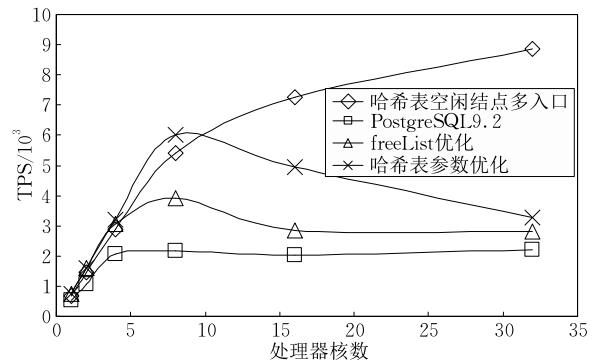
图 7 不同的缓冲区管理策略下,系统的扩展性
