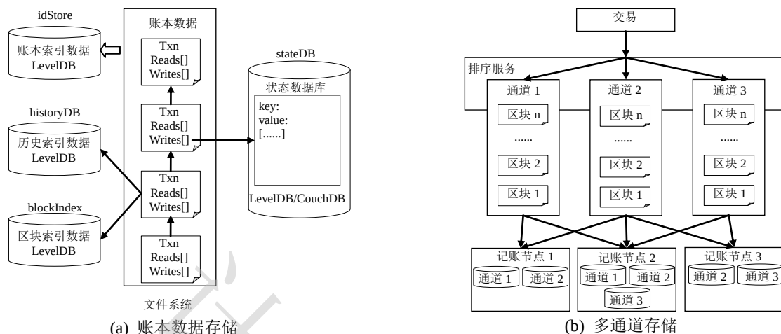
图 6 超级账本的分布式存储结构
