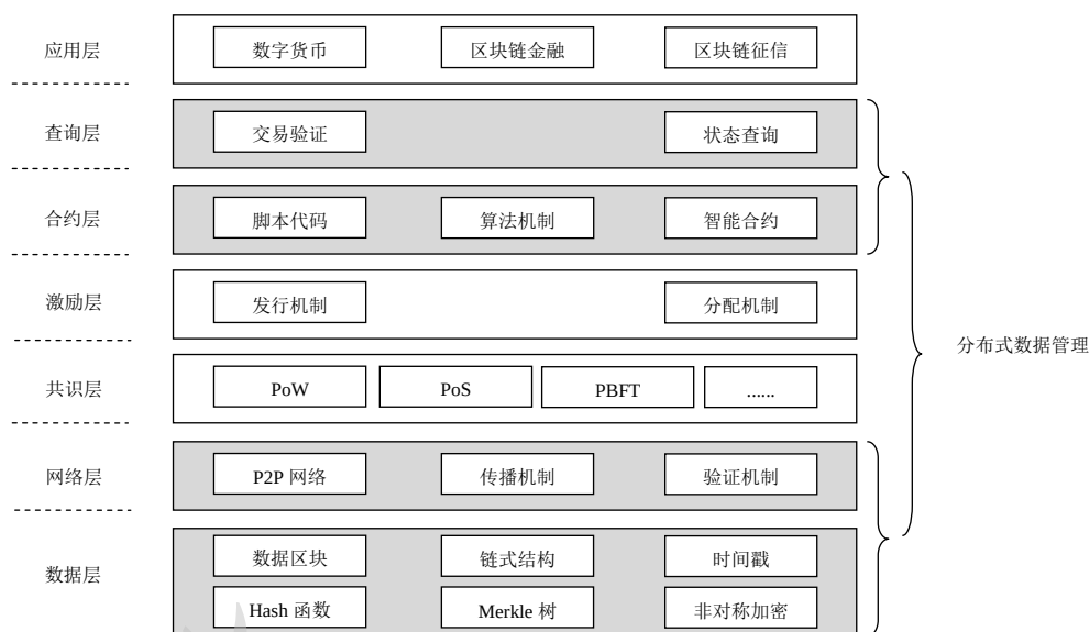
图 1 区块链系统的架构模型
