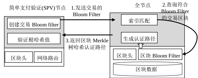
图7 简单支付验证的分布式查询处理
