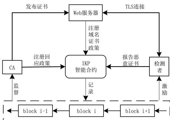
图 15 IKP 架构图 [76]
