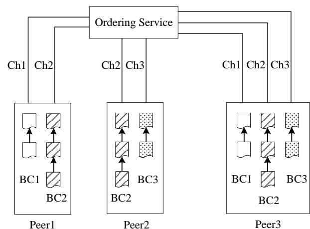
图7 Hyperledger Fabric 多通道
