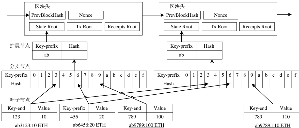
图3 Merkle Patricia 树
