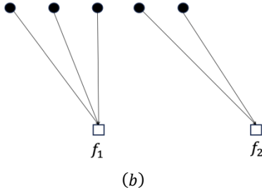
图 2 (a) 开设设施 f_1 时用户的连接方式；(b) 开设设施 f_1 与 f_2 时用户的连接方式，其中， \tau(f_2) = 2 。可以看出，在该实例中增加开设设施数量会增大某些用户的连接费用。
