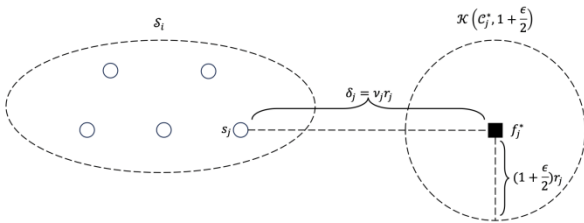
图 9 引理 9 证明中的基本符号
