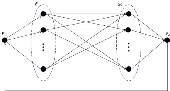
图 7 最小费用循环流问题实例
