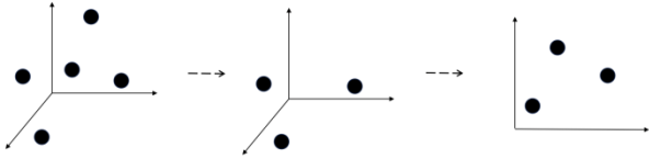
图 8 基于引理 6 和推论 1 的降维方法
