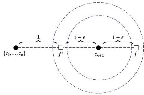
图 3 实例 (\{c_1, \dots, c_{n+1}\}, \{f^*, f\}, 1, \tau)
