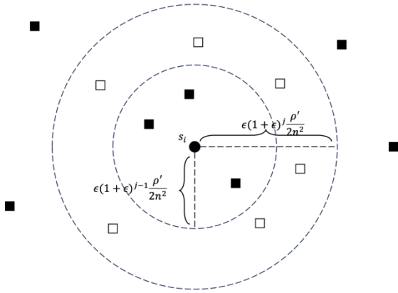
图5 集合 \mathcal{L}(i, j) 中的设施
