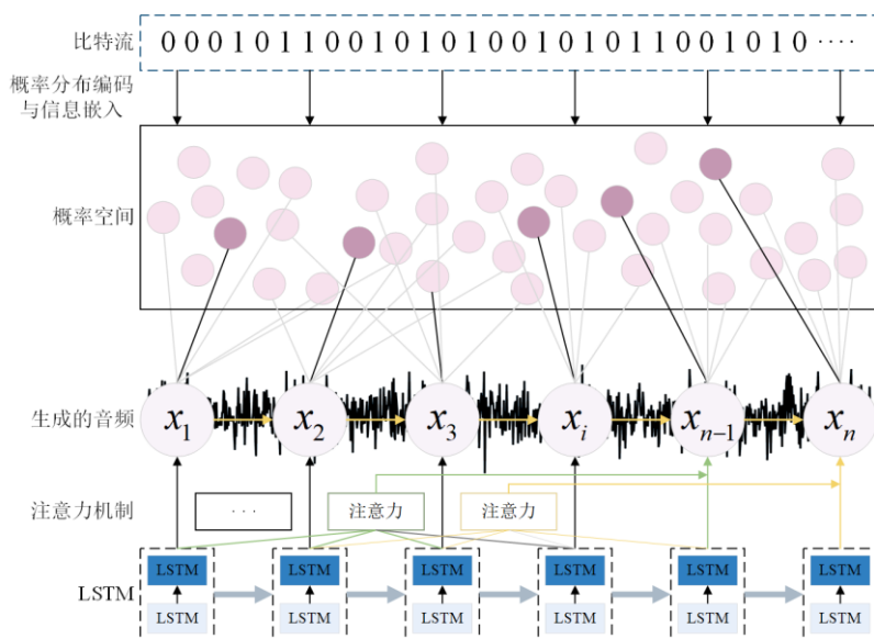
图 15 AAG-Stega 隐写模型
