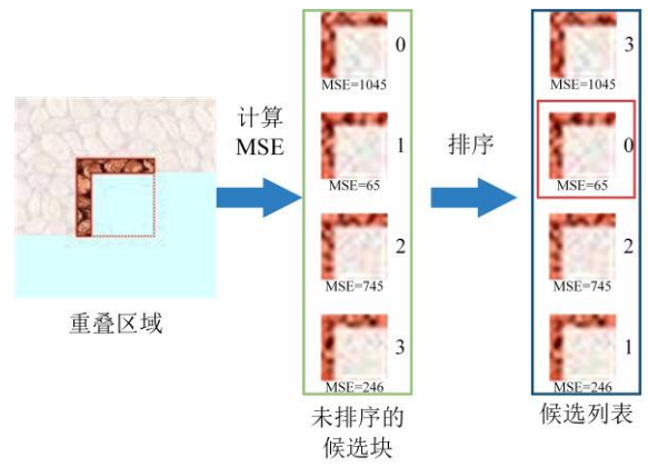
图6 Wu 等 [62] 候选图像块列表的建立
