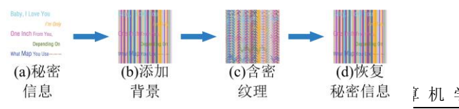
图5 stego-texture 隐写模型
