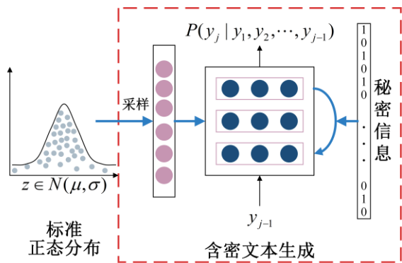
图14 VAE-Stega 隐写模型
