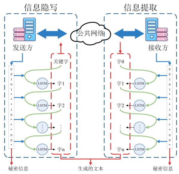
图 13 RNN-Stega 隐写模型
