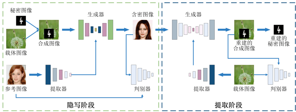
图 10 Li 等[74]隐写模型
