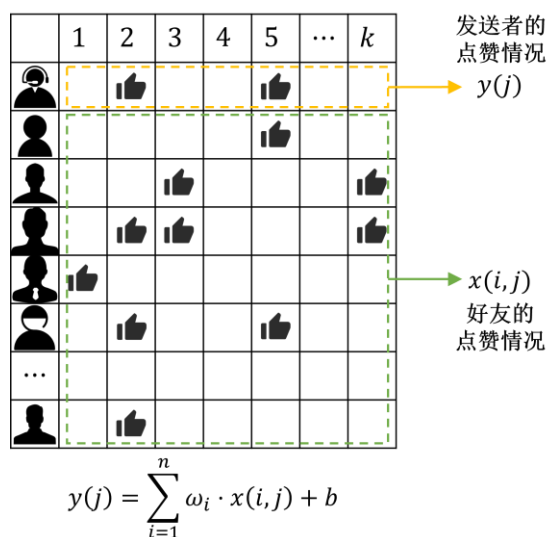
图 16 Hu 等 [113] 提出的用户行为相关性模型
