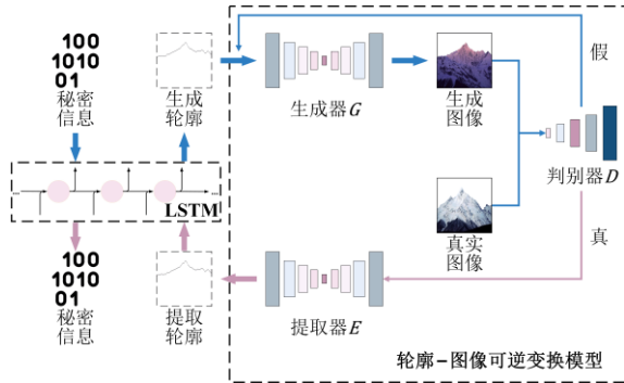
图 7 Zhou 等[66]隐写模型
