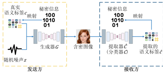
图 8 SSS-GAN 隐写模型
