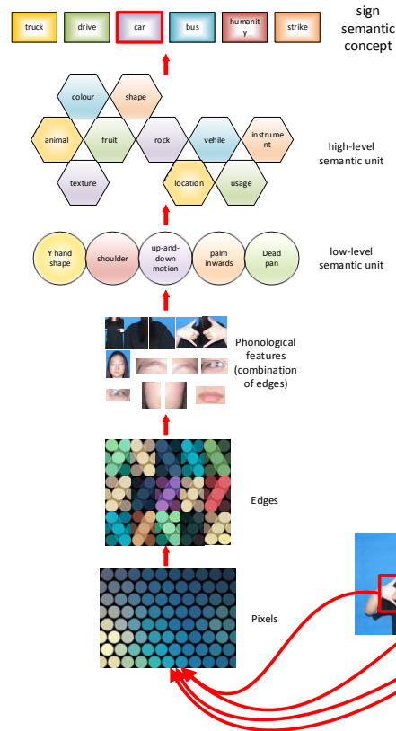
图 9 手语认知计算架构
