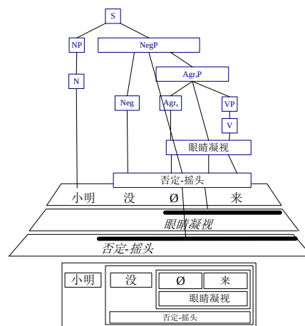
图6 3D 语法树
