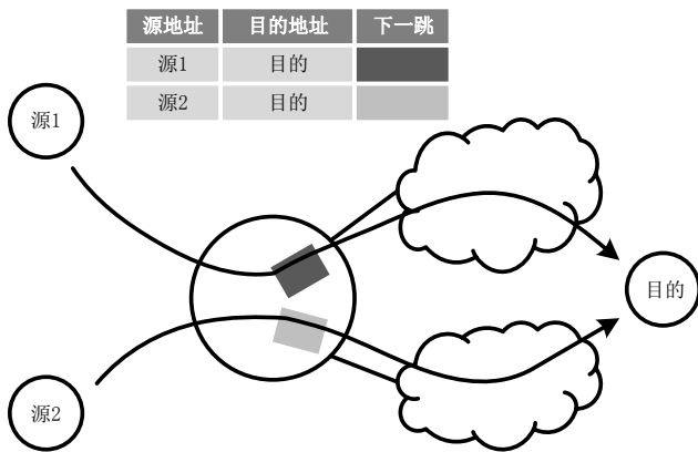
图 4 基于二维路由的转发表示意图
