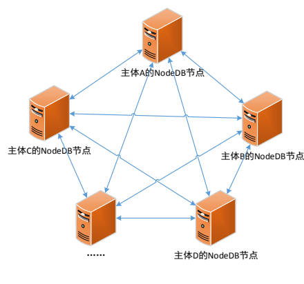
图 7 全网 NodeDB 架构
