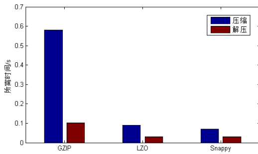
图 10 压缩算法解压、压缩效率
