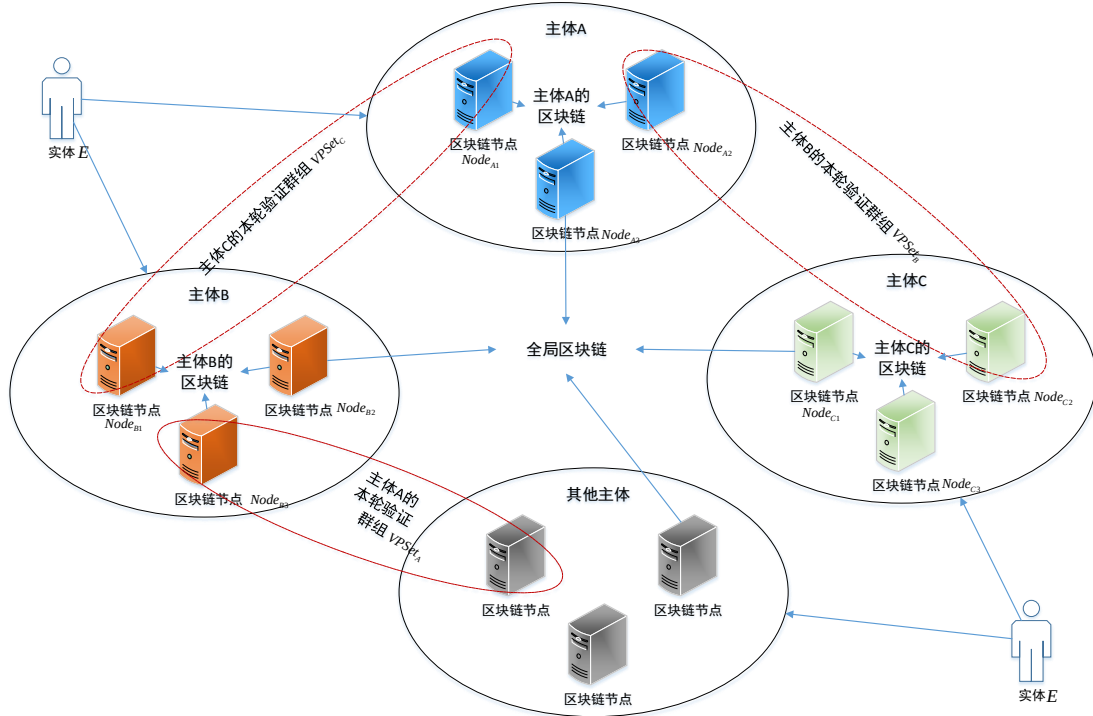
图 1 许可链多中心动态共识机制架构
