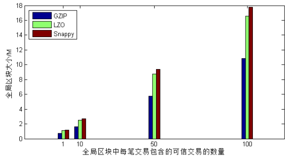
图 9 全局区块链压缩量对比
