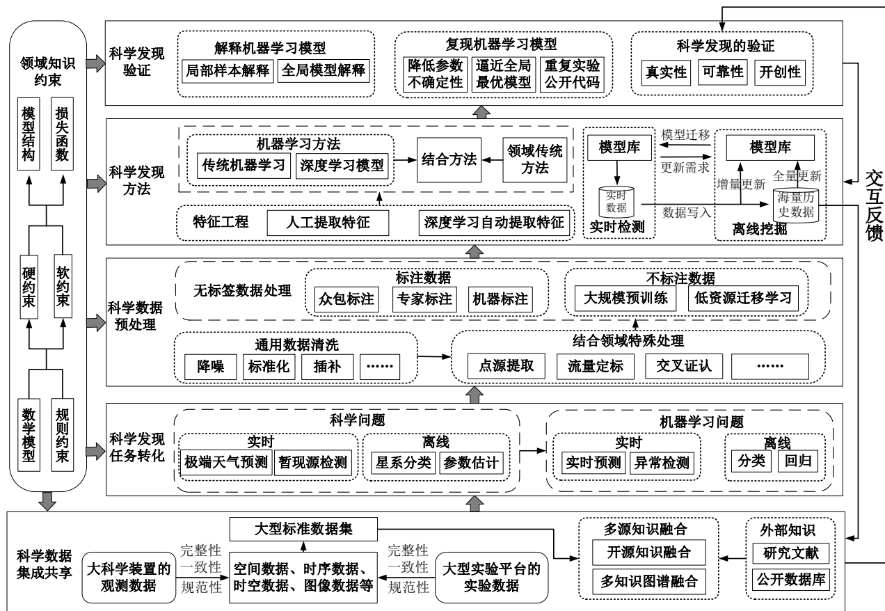
图1 基于机器学习的智能科学发现研究框架
