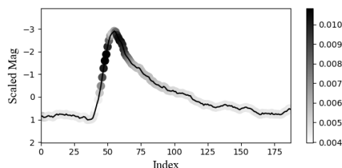
图3 FCN 正确分类为耀发样本的 CAM 热力图
