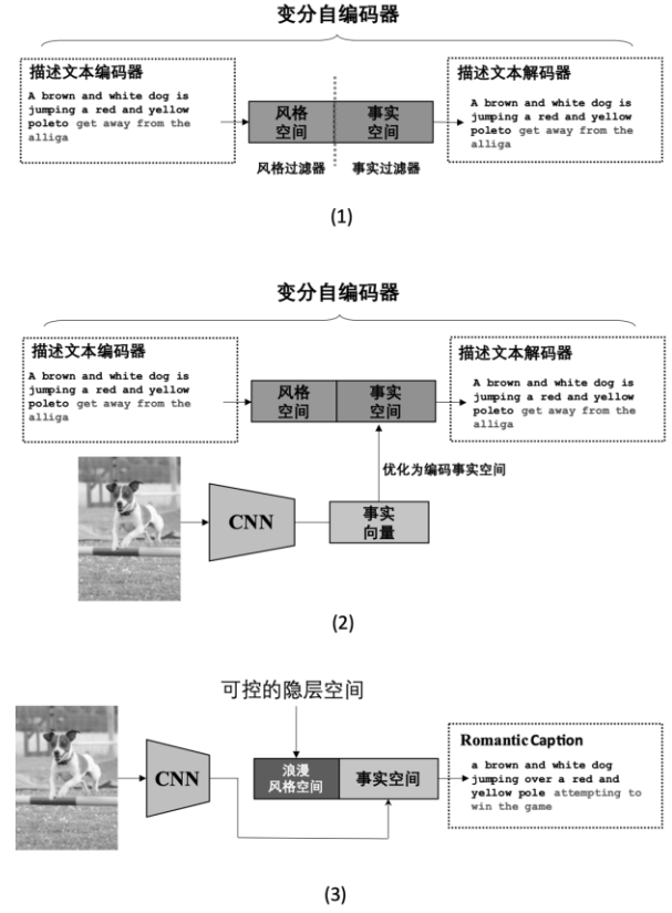
图 6 D-Captions 模型。(1) 利用过滤器来学习描述文本隐层空间的解纠缠表示。(2) 训练图像编码器编码事实空间。(3) 对图像编码器和变分编码器中的解码器进行联合微调。在图示例子中, 模型利用从变分自编码器中得到的浪漫风格表示和从图像编码器中得到的事实表示来生成浪漫风格的描述文本。
