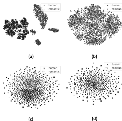
图3 t-SNE图: (a) D-Captions 模块解纠缠的风格空间, (b) D-Captions 模块解纠缠的事实空间, (c) D-Images 模块解纠缠的风格空间, 以及 (d) D-Images 模块解纠缠的事实空间。
