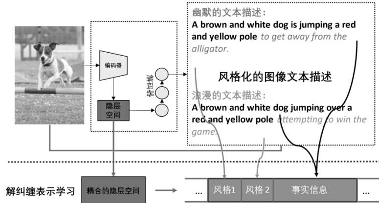
图 1 一个风格化图像文本描述生成的例子。在图像上半部分的端到端模型中，隐层空间的信息的含义几乎无法被人类所理解。而图像下半部分通过解纠缠表示学习能一定程度提升对跨媒体模型的耦合的隐层空间的可控性和可解释性。
