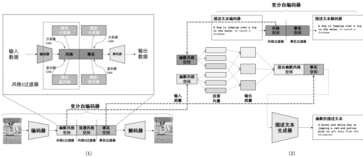
图2 模型概览。(1) 对图像和描述文本的隐层空间表示进行解纠缠处理。(2) 将之前从图像中和描述文本中获得的跨媒体风格向量进行聚合，并结合事实信息利用描述文本生成器生成风格化的图像描述。
