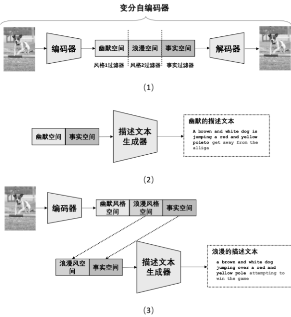
图 5 D-Images 模型。(1) 利用过滤器学习图像隐层空间的解纠缠表示。(2) 使用对应风格的描述文本和风格及事实表示训练描述文本生成器。(3) 对变分自编码器的编码器和描述文本生成器进行联合微调。
