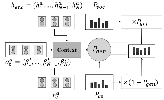
图 3 生成答案的指针网络
