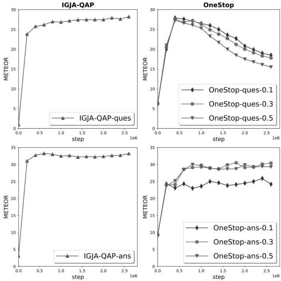
图 5 IGJA-QAP 和 OneStop 在训练过程中问题生成和答案生成的指标变化曲线。图中'ques'和'ans'分别待变问题生成和答案生成。左栏表示在 IGJA-QAP 上的变化曲线, 右栏表示在 OneStop 上的变化曲线
