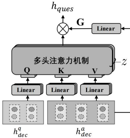
图 4 答案引导的多头门机制
