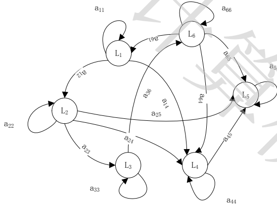
图3 用户在六个状态下移动的马尔可夫链模型
