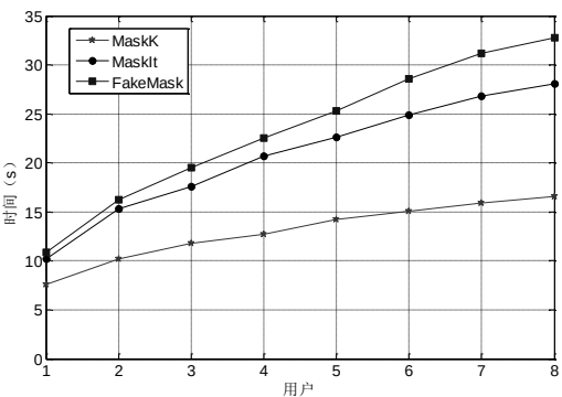
图 13 位置个数不同时三种方法计算抑制发布概率向量所需时间的对比图
