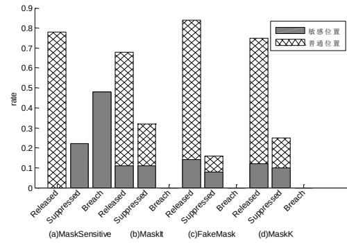
图 9 四种方法隐私检验结果的柱状图
