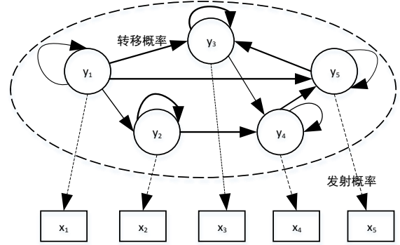
图4 某用户位置发布的 HMM
