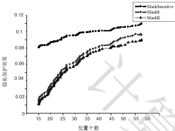
图 10 基于 Forward-Backward 算法的攻击模型下三种方法的隐私保护机制的安全性 ( \delta=0.1 )
