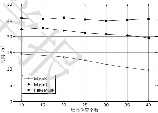
图 14 敏感位置个数不同时三种方法计算抑制发布概率向量所需时间
