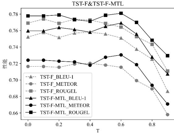
图 2 以 CoQA 为源领域数据集，不同阈值下，TST-F 和 TST-F-MTL 在 TweetQA 开发集的性能对比。
