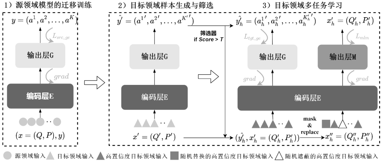
图 1 迁移自训练-筛选器-多任务学习 (TST-F-MTL) 模型框架
