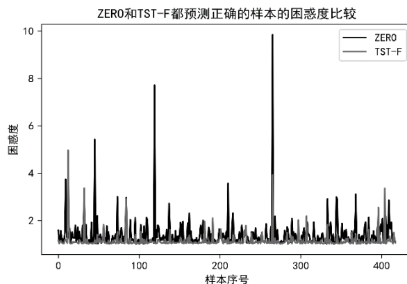
图 4 TweetQA 开发集在 ZERO 和 TST-F 上预测都正确的 418 条样本的困惑度对比
