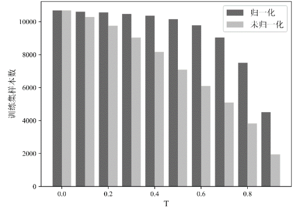
图3 以 SQuAD 为源领域数据集, 不同阈值下, 归一化与未归一化筛选的 TweetQA 训练集样本个数。
