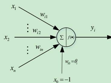
图 1 神经元的 M-P 模型示意图
