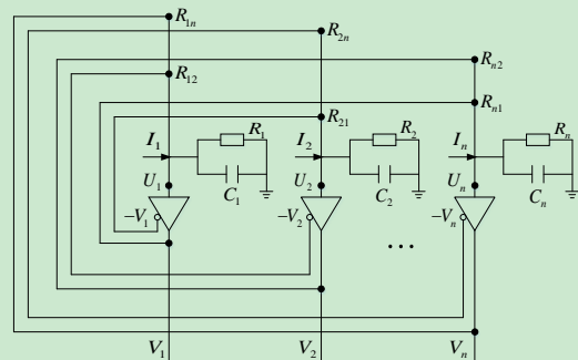
图 2 典型的 Hopfield 网络模型
