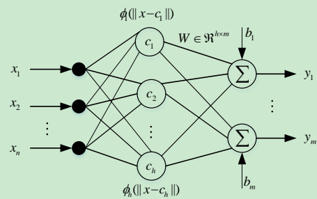
图 5 RBF 神经网络基本结构示意图
