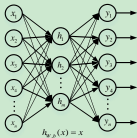
图 6 自编码器示意图
