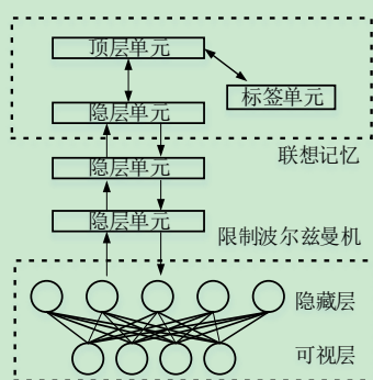
图 9 DBN 结构示意图
