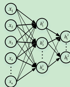
图 8 栈式自编码器示意图
