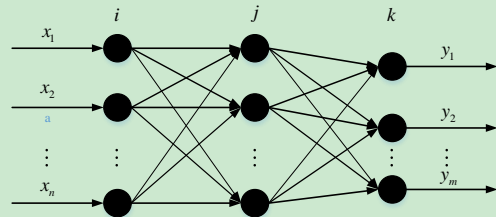
图 4 三层 BP 网络示意图
