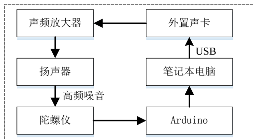
图4 检测陀螺仪共振频段的流程图
