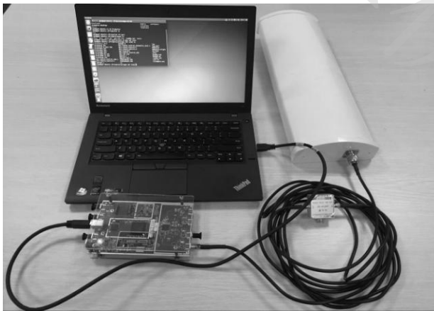
图 6 GPS 欺骗系统设备图（包括主机、USRP 和天线）
