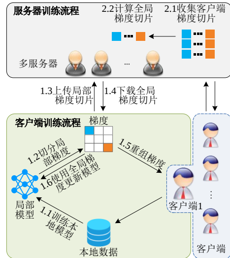
图8 FGFL 拓扑结构
