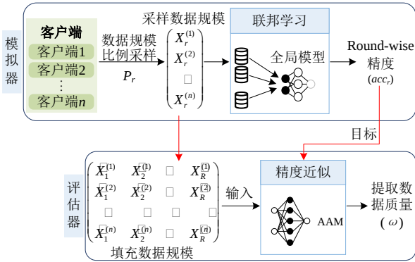
图3FedCCEA框架
