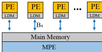
图 4 典型 PRAM 多核并行计算模型
