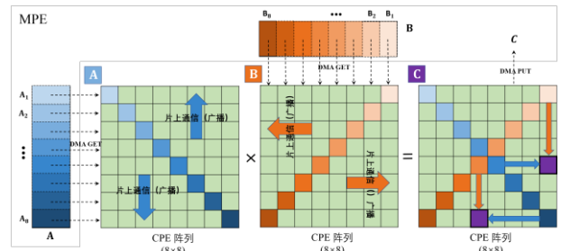
图5 矩阵乘并行计算流程示意图
