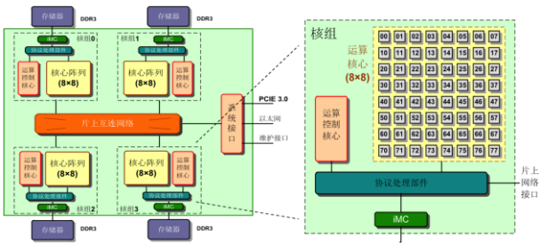
图1 “申威 26010”异构众核处理器架构图
