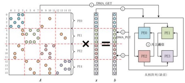
图 6 SPMV 并行计算流程示意图
