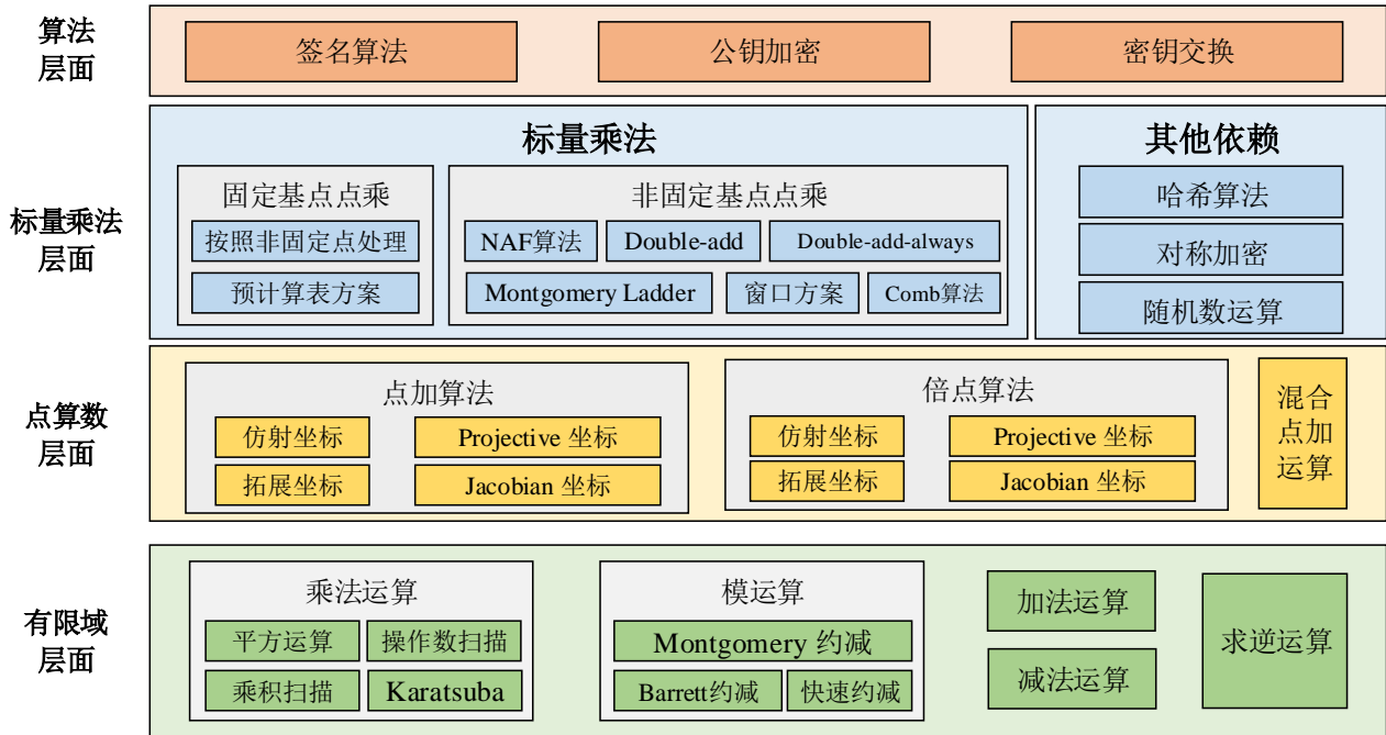
图 3 椭圆曲线密码算法架构
