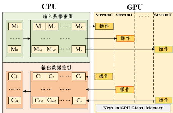
图2 基于 GPU 平台的密码计算模型
