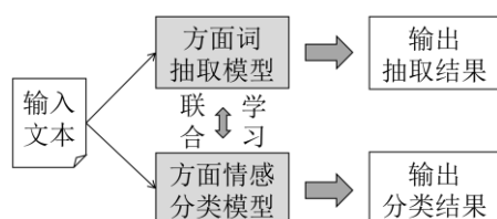
图 12 基于联合学习的方面-情感对抽取
