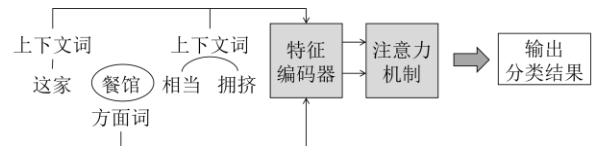
图 7 基于注意力机制的方面情感分类
