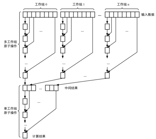
图 10 TensorFlow 中多工作组原子操作计算示意图
