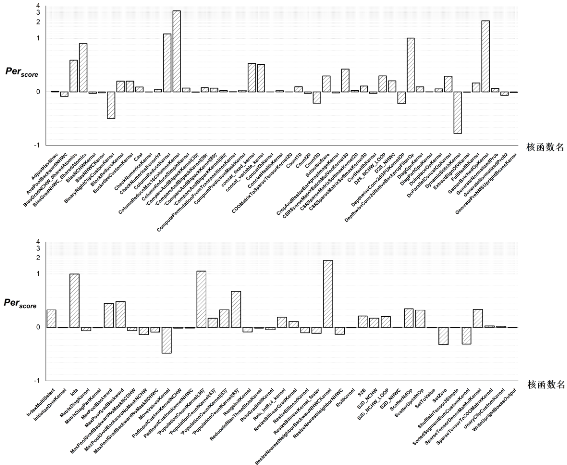
图 18 OpenCL 核函数与对应 CUDA 核函数性能对比图
