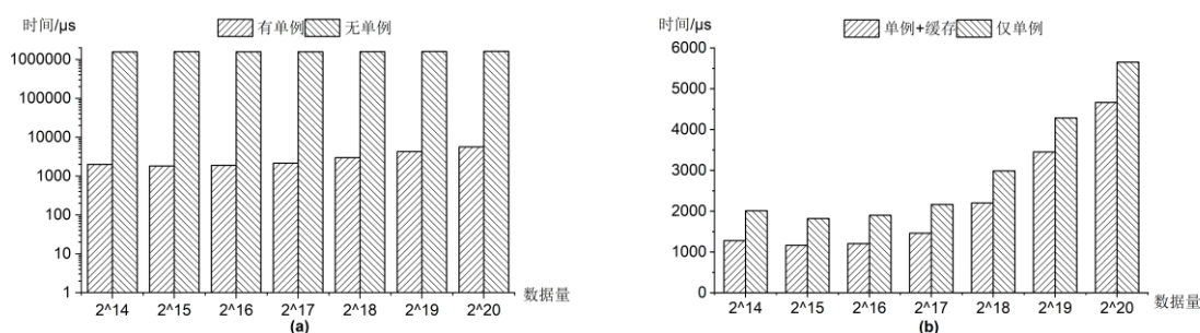
图 20 不同输入数据规模下使用不同优化策略核函数性能对比: (a) 使用单例进行优化与未优化时核函数在不同输入数据规模下的性能对比; (b) 使用单例+缓存的组合优化模式与仅使用单例优化时核函数在不同输入数据规模下性能对比
