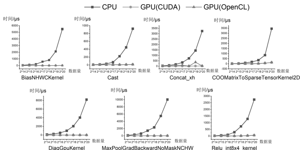
图 19 7 种典型核函数在不同输入数据规模下使用 CPU、GPU(OpenCL)、GPU(CUDA)运算时间的对比
