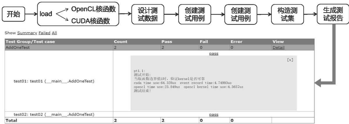
图 17 核函数测试流程及测试报告样例
