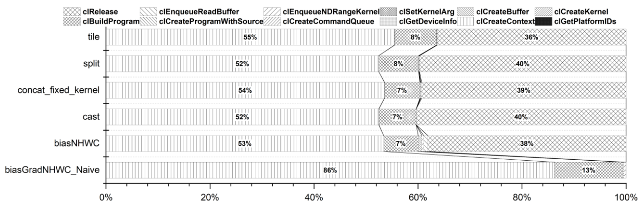
图8 典型 OpenCL 核函数代码中 OpenCL 接口执行时间占比统计
