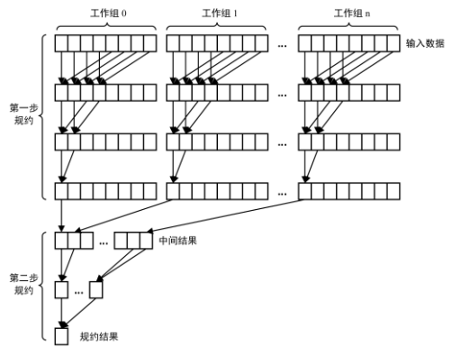
图 11 两步规约计算示意图
