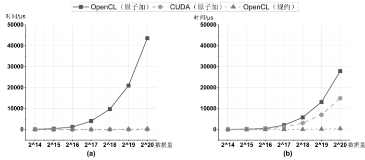
图 21 规约算法替换原子加操作的优化效果: (a) 输入数据类型为 float32 时算子使用 OpenCL 原子加、CUDA 原子加以及 OpenCL 规约算法在不同数据规模下的性能对比; (b) 输入数据类型为 double 时算子使用 OpenCL 原子加、CUDA 原子加以及 OpenCL 规约算法在不同数据规模下的性能对比。
