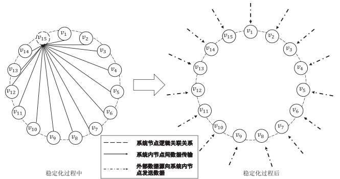
图2 无写扩展过程的系统拓扑模型变化
