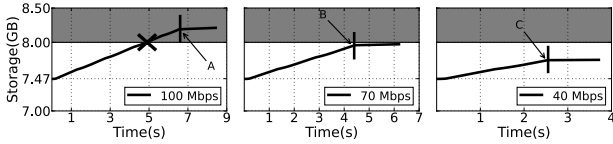
图7 时间限制：不同写入速率 \lambda (灰色区域为失效区，竖线标志位置为稳定化过程中的累积写入被处理完成的時刻)
