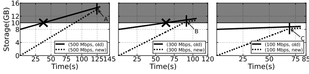
图3 存储空间限制：不同写入速率 \lambda (灰色区域为失效区，竖线标志位置为稳定化过程结束的時刻)
