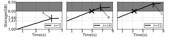
图8 时间限制：不同系统规模 N (灰色区域为失效区，竖线标志位置为稳定化过程中的累积写入被处理完成的時刻)
