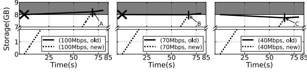
图5 带宽限制：不同写入速率 \lambda (灰色区域为失效区，竖线标志位置为稳定化过程结束的時刻)
