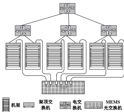
图1. c-Through 网络架构
