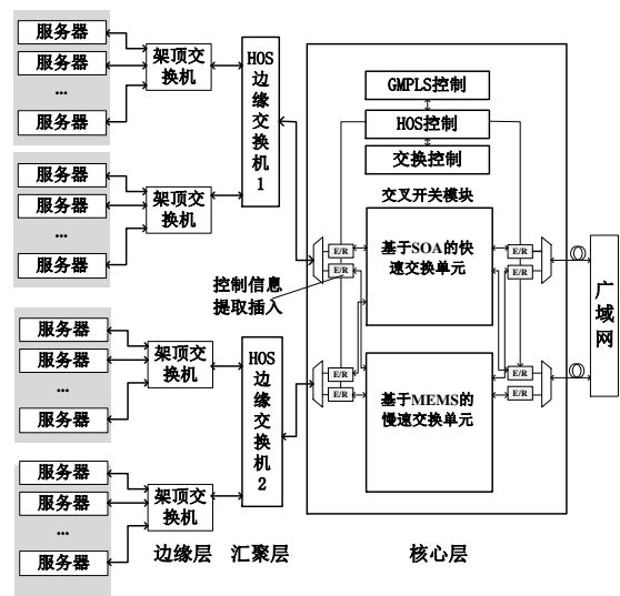
图13. HOS 混合全光交换架构
