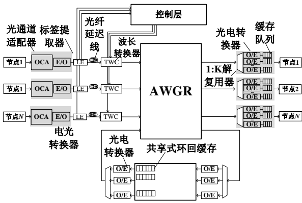
图6. DOS 全光互连架构
