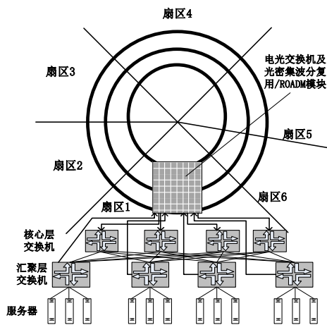
图14. FISSION 全光互连架构
