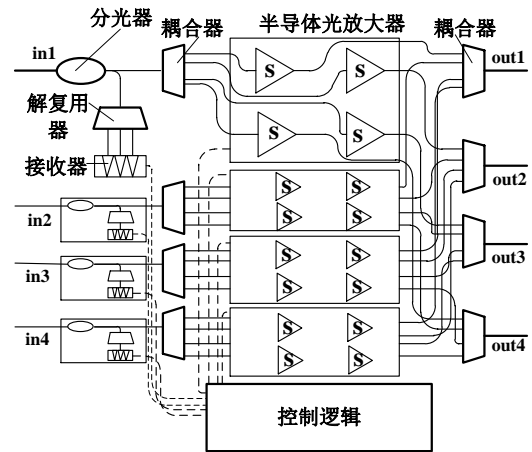
图12. 基于 SOA 的混合交换架构
