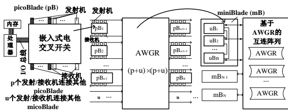
图10. 基于 AWGR 的分层架构
