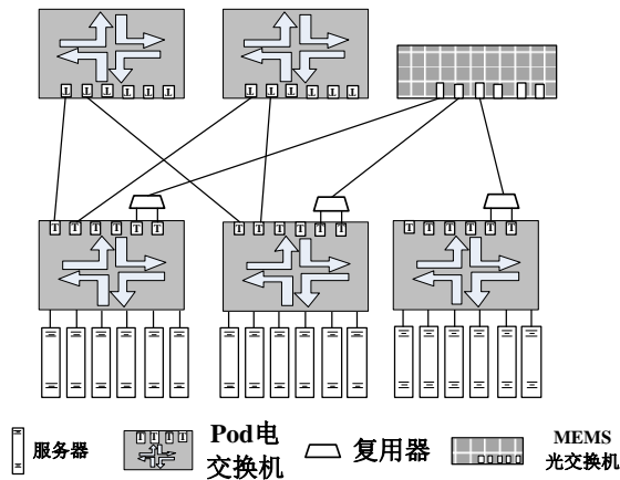
图2. Helios 网络架构
