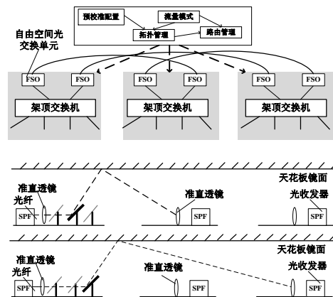
图15. 自由空间光网络 FireFly 架构
