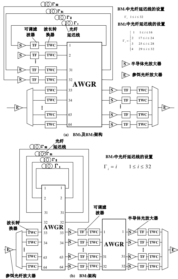
图7. 基于光纤延迟线的 AWGR 环回架构
