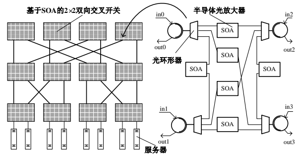
图11. 基于 SOA 的 fat tree 网络
