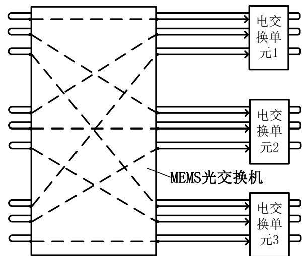
图3. 混洗-交换网络架构
