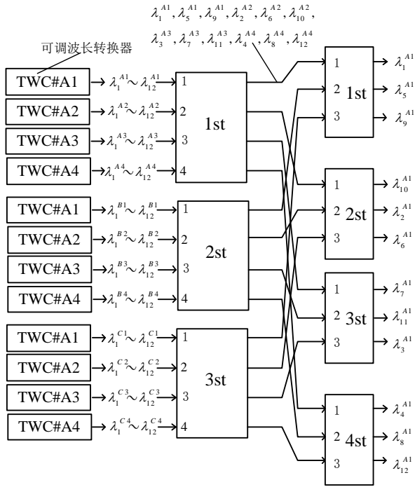
图8. 两级 AWGR 架构
