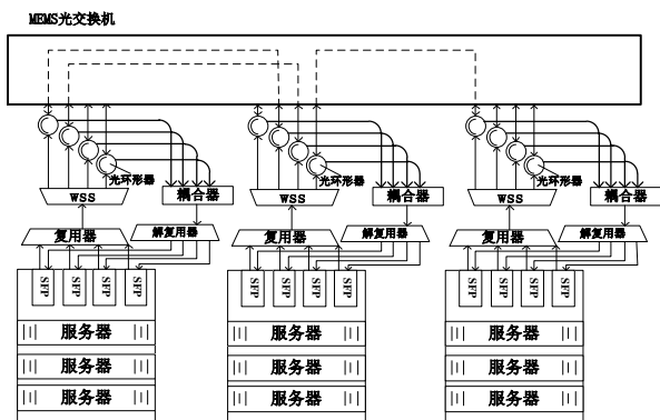
图5. Proteus 全光交换架构
