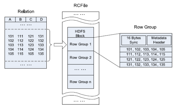
图 2 RCFile 数据存储结构示例[44]
